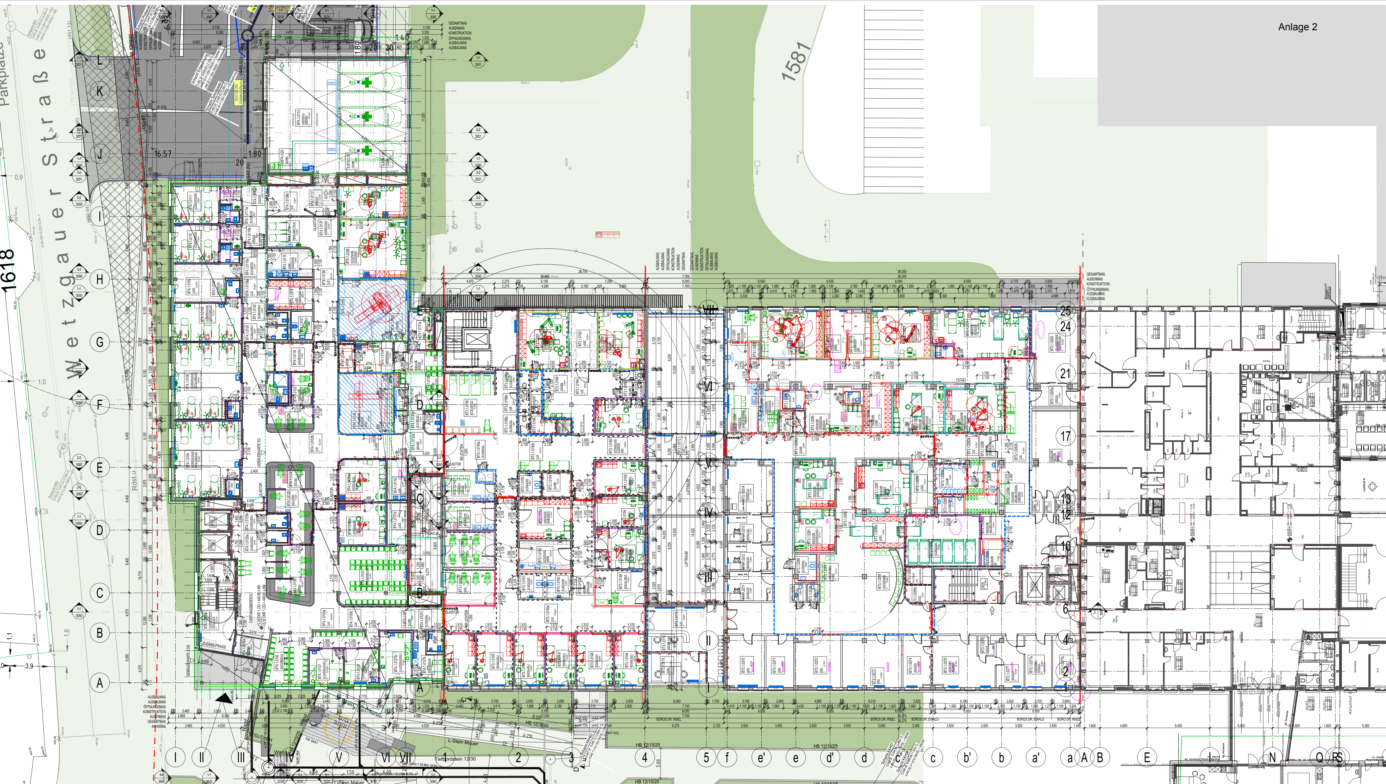
NEUBAU ZENTRALE NOTAUFNAHME BT4
