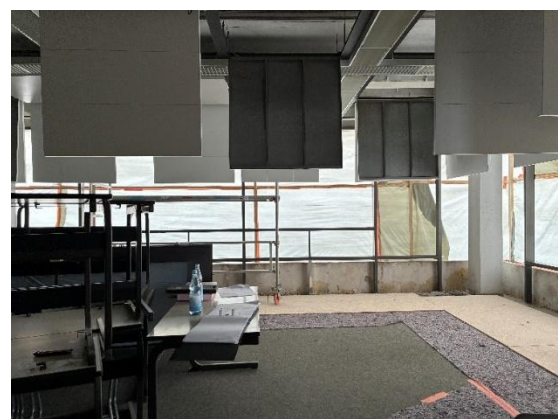
Beginn der neuen Fassadenkonstruktion
