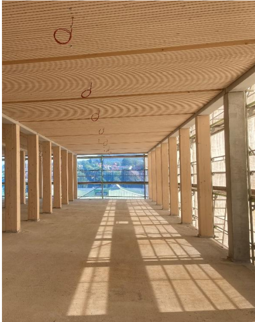
Innenansicht mit Holzstützen und Holzbetonverbunddecken
