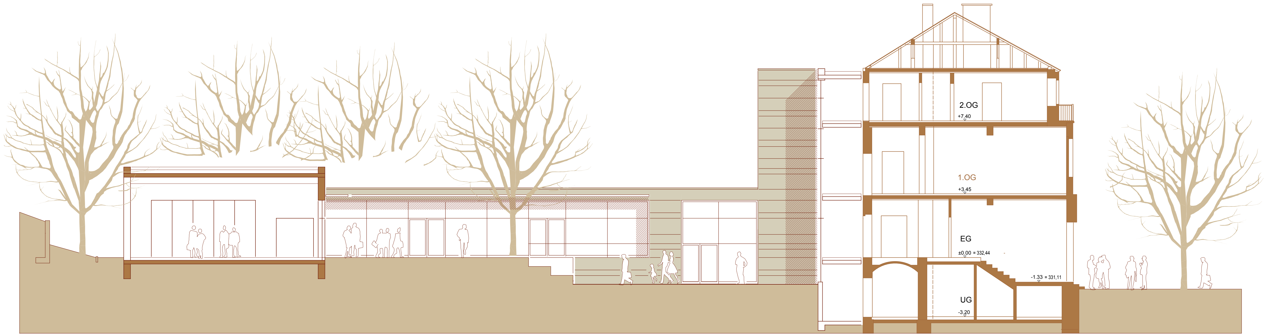
Pausenhof - Schnitt Universalraum Pausenhof Vorfahrt 2 Südwest - Ansicht
