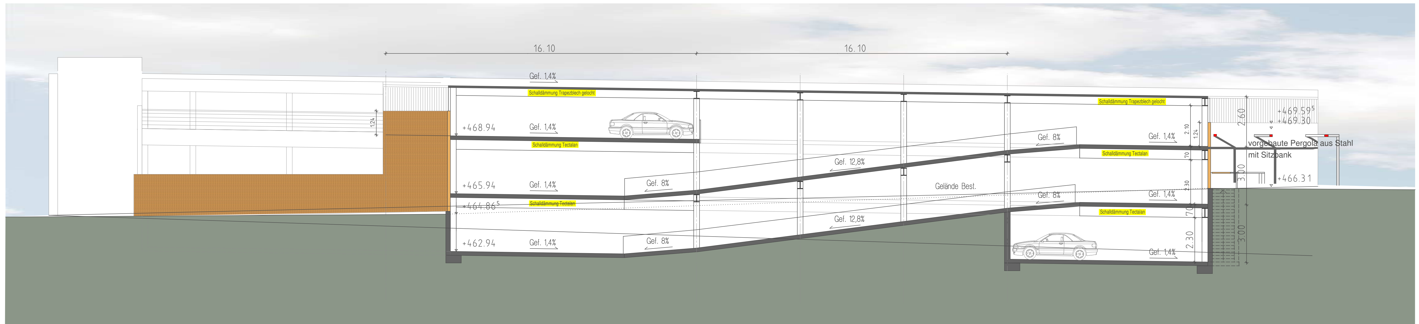
SCHNITT A - A
