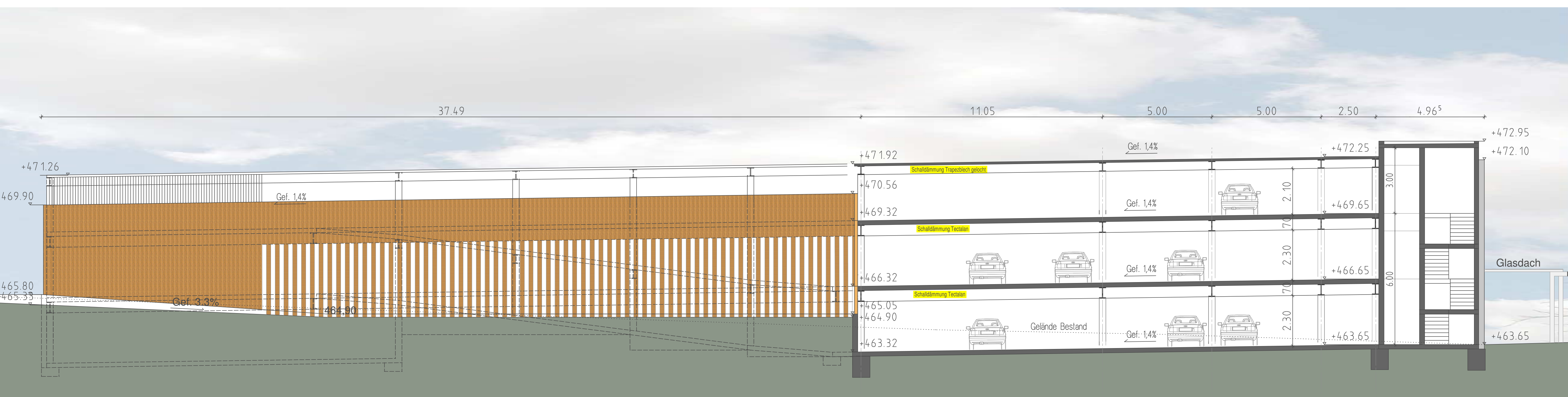
SCHNITT C - C / ANSICHT NORDOST
