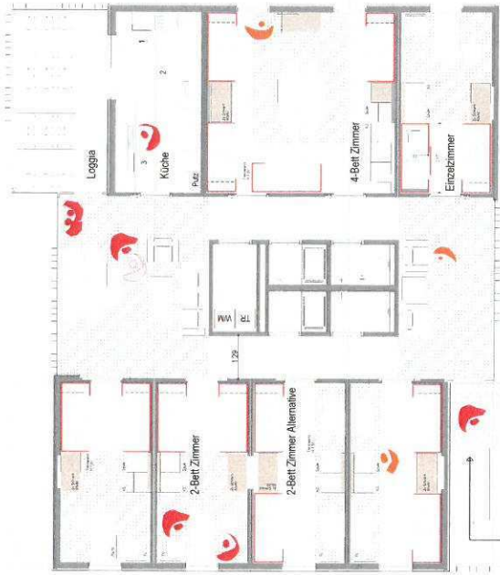
Grundriss Wohneinheit M1/50
