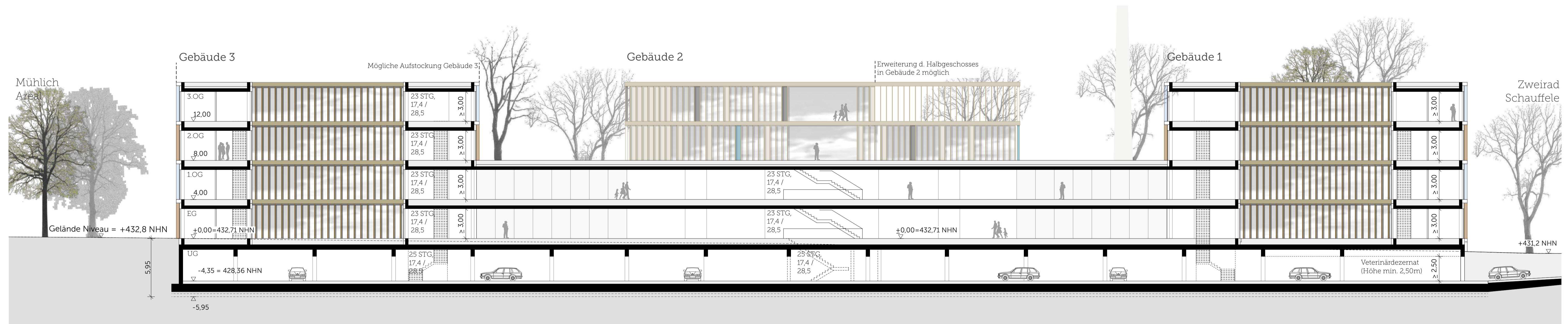
Schnitt A- A
